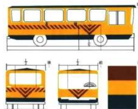
公私立各級學校(含幼稚園、托兒所)校車顏色及標誌標準圖
